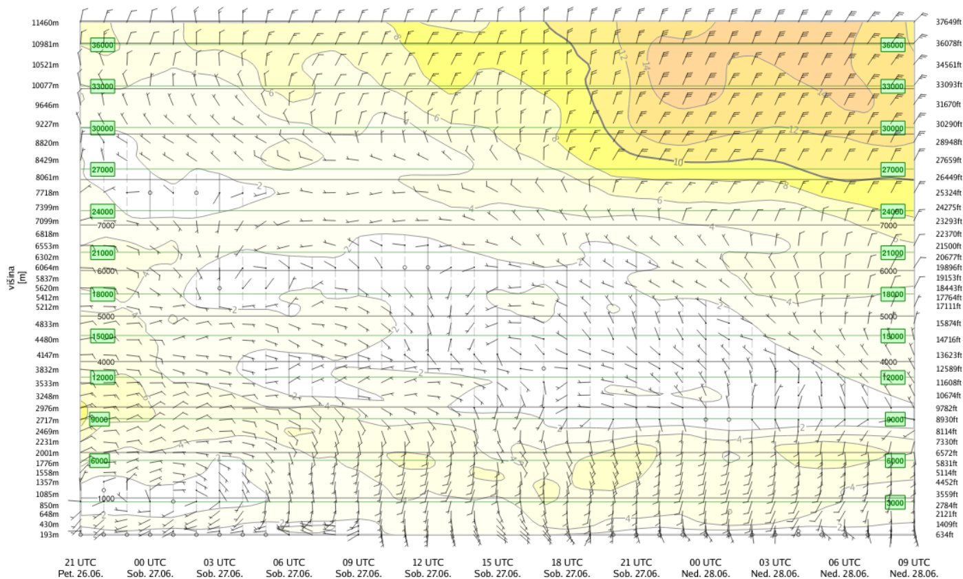
VERTIKALNI ČASOVNI PRESEK 26.06.2026 21:00 - 28.06.2026 09:00 Murska Sobota Napoved modela ALADIN/SI ECDA: hitrost vetra (m/s)
